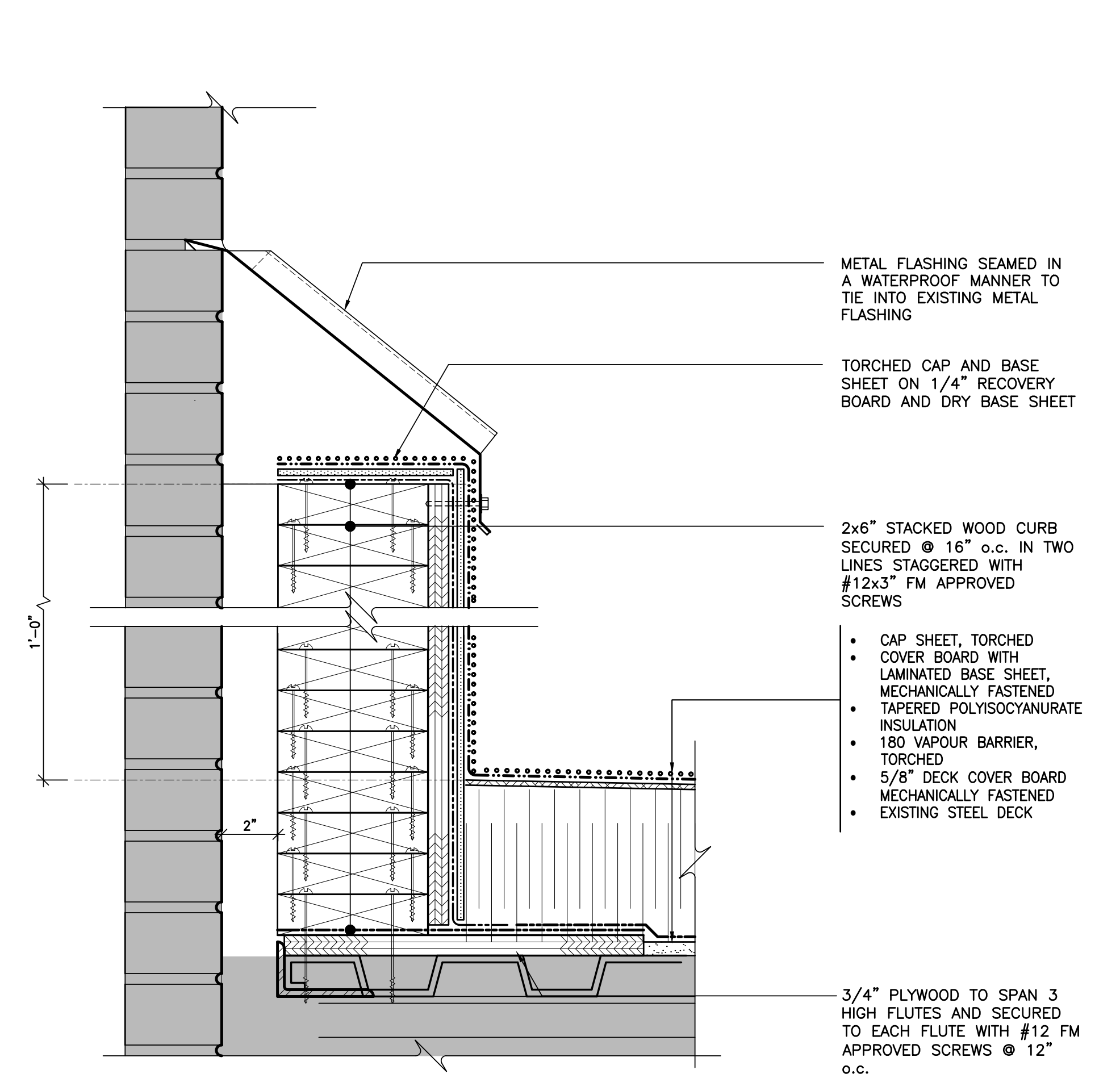
5 A-2 SECTION DETAIL CHIMNEY CURB SCALE: 3" = 1'-0"
