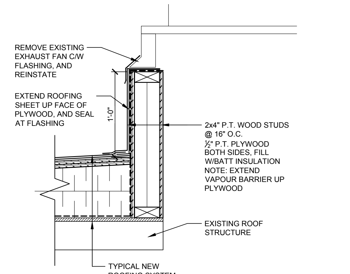
5 FAN CURB DETAIL A-101 1-1/2"=1'-0"
