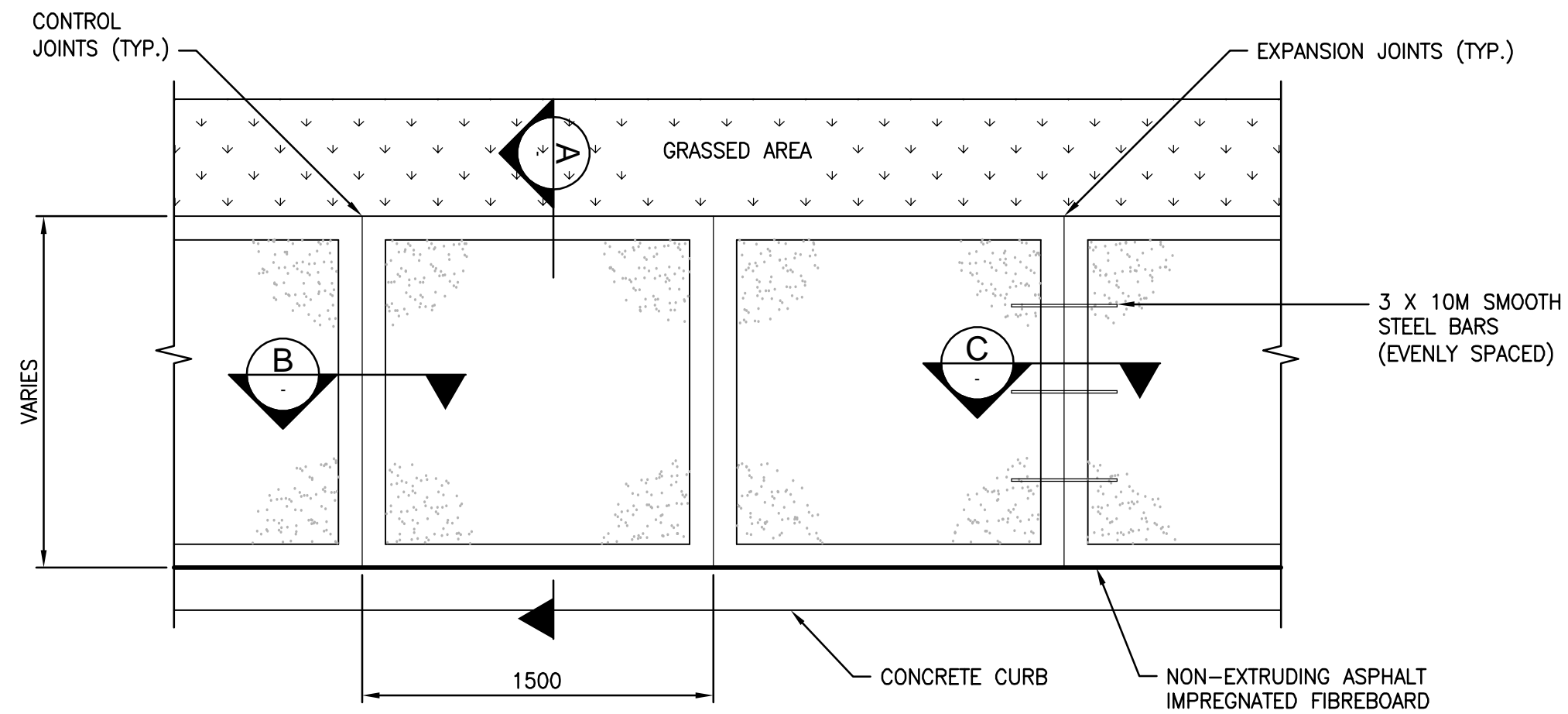
SIDEWALK PLAN N.T.S.
